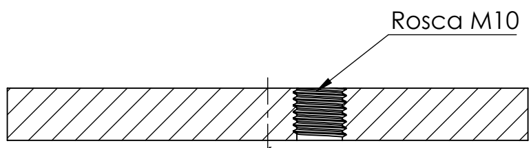
SECCIÓN A-A ESCALA 1 : 1
